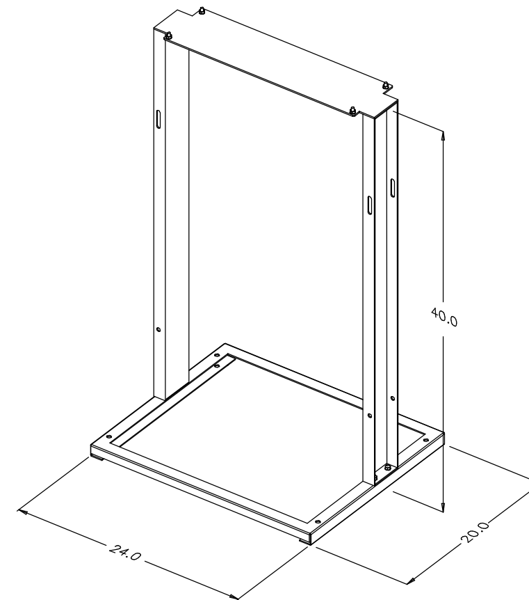
OPTIONAL STAND
